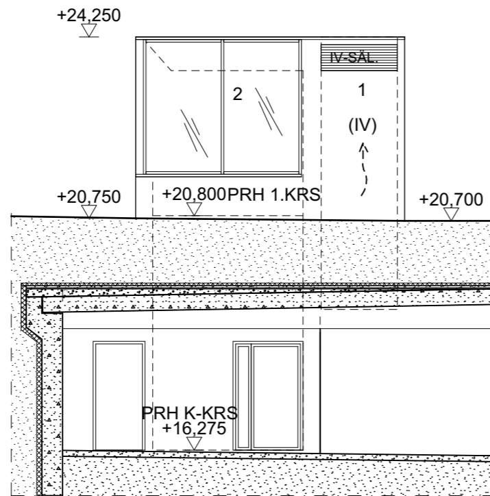
JULKISIVU LOUNAASEEN/LEIKKAUS
